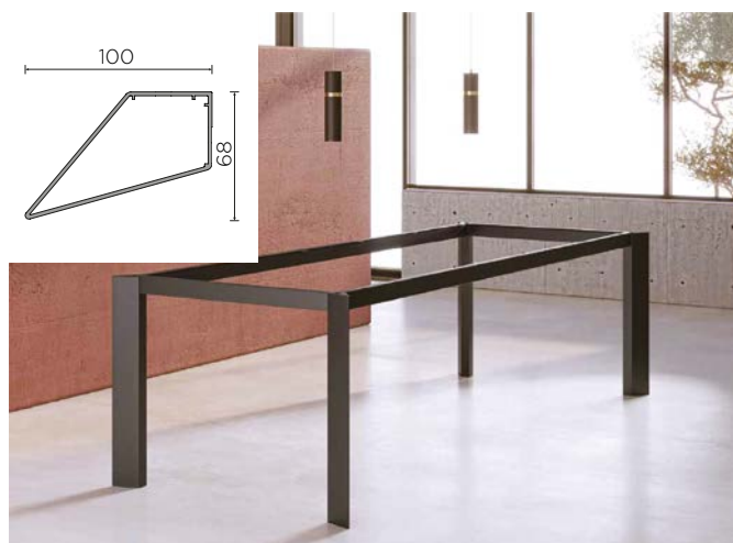
B4 (profil nog: 100 x 68 mm)
