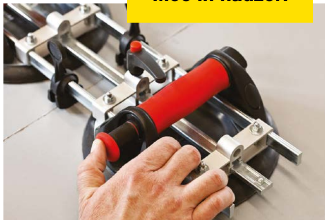
Ročna vakuumska črpalka: Omogoča nadzorovanje tlaka in doseganje vpenjalne sile do kar 1200 N.
