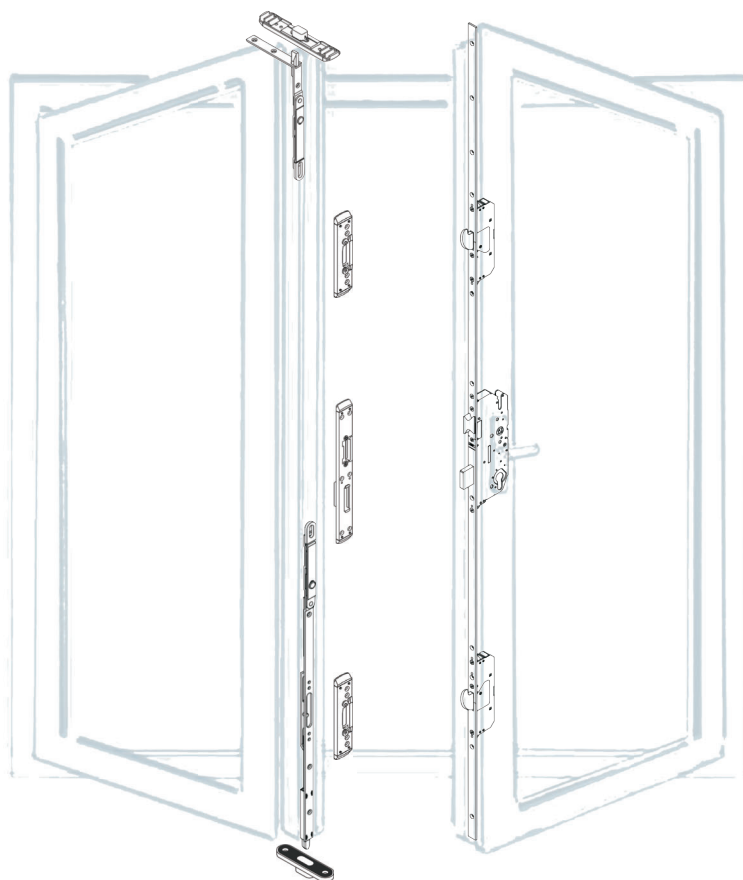
Dvokrilna PVC vrata s pettočkovno ključavnico
