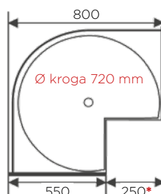
žični vrtljivi sistem
