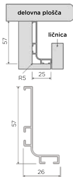
kapica L za zunanji profil
