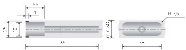
shema vrtnja za police debeline nad 30 mm
