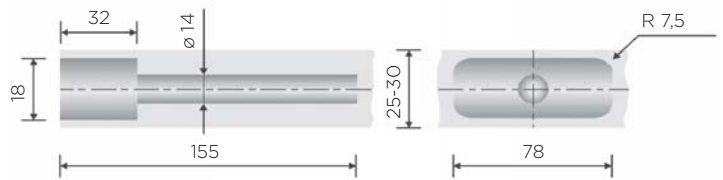
shema vrtnja za police debeline 25-30 mm
