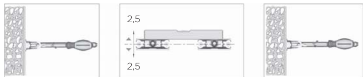
vertikalna nastavev
