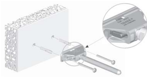
pritrnitev na betonsko steno
