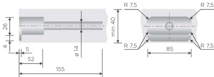
shema vrtanja
