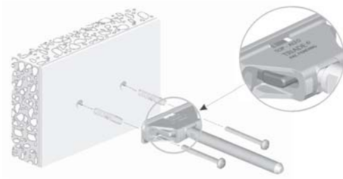
pritrnitev na betonsko steno
